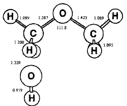
(d) \text{CH}_3\text{OCH}_2\text{O}
